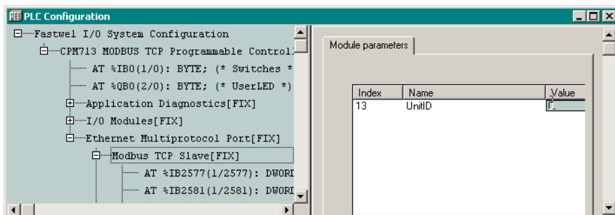
Рис. 3. Параметр UnitID сервера протокола MODBUS
