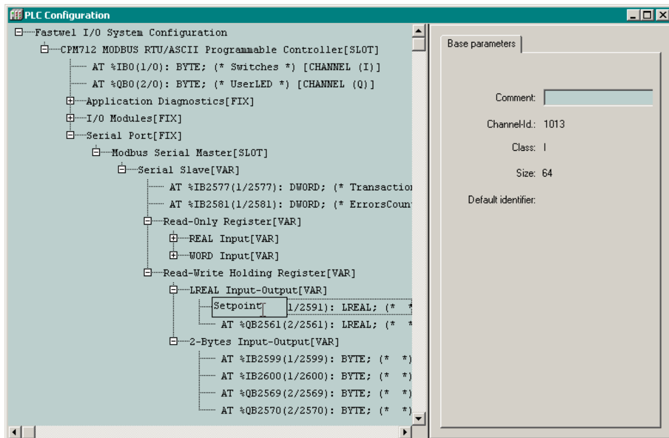
Рис. 11. Создание символических ссылок
