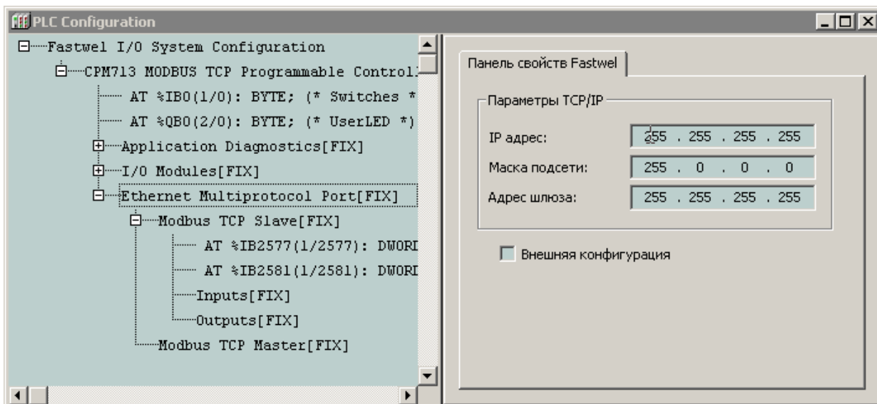
Рис. 2. Элемент конфигурации для настройки параметров TCP/IP
