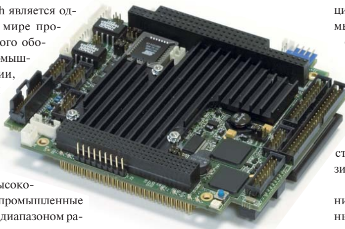
Рис. 1. Внешний вид одноплатного компьютера FASTWEL™ CPC304
